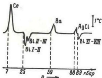
Рис. 2. Сводная термограмма для различных веществ
